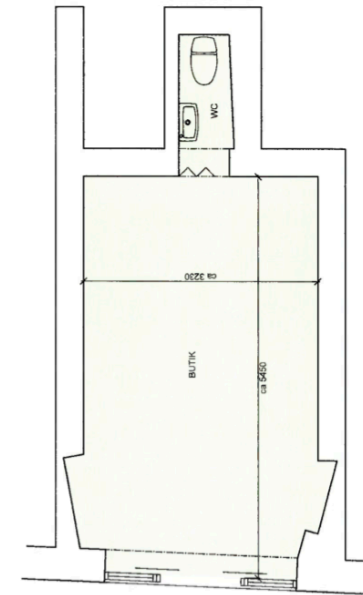
Plan 1 (Butik) skala 1:50
